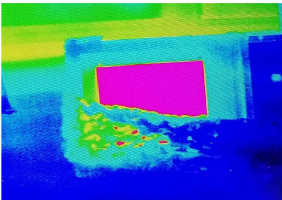
Termogramma in "falsi colori" rilevata da sensore infrarosso in cui la rete di mascheramento inibisce la visione della radiazione termica generata dal calore della piastra
